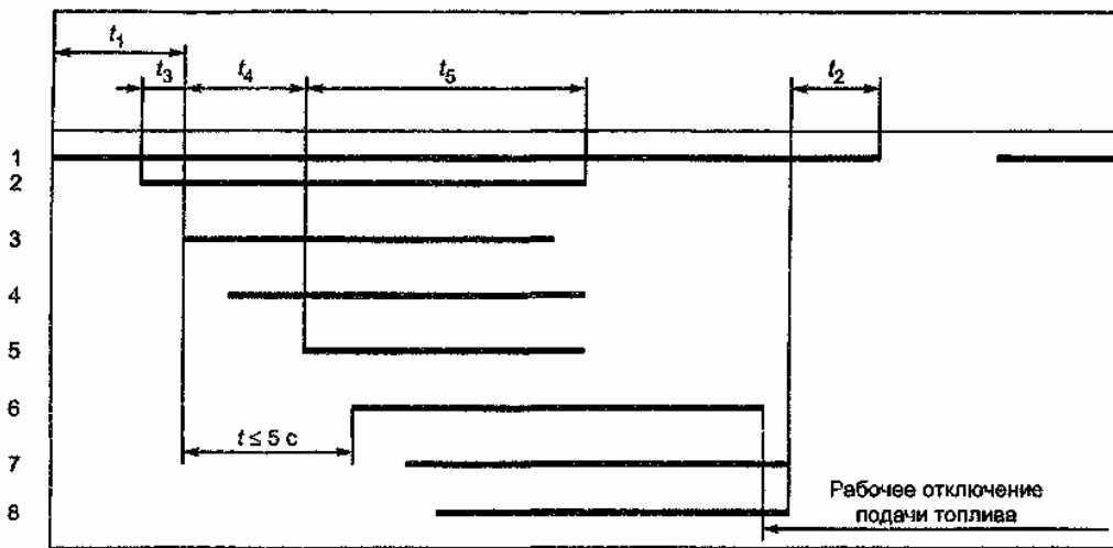
Диаграммы с защитным отключением при розжиге
